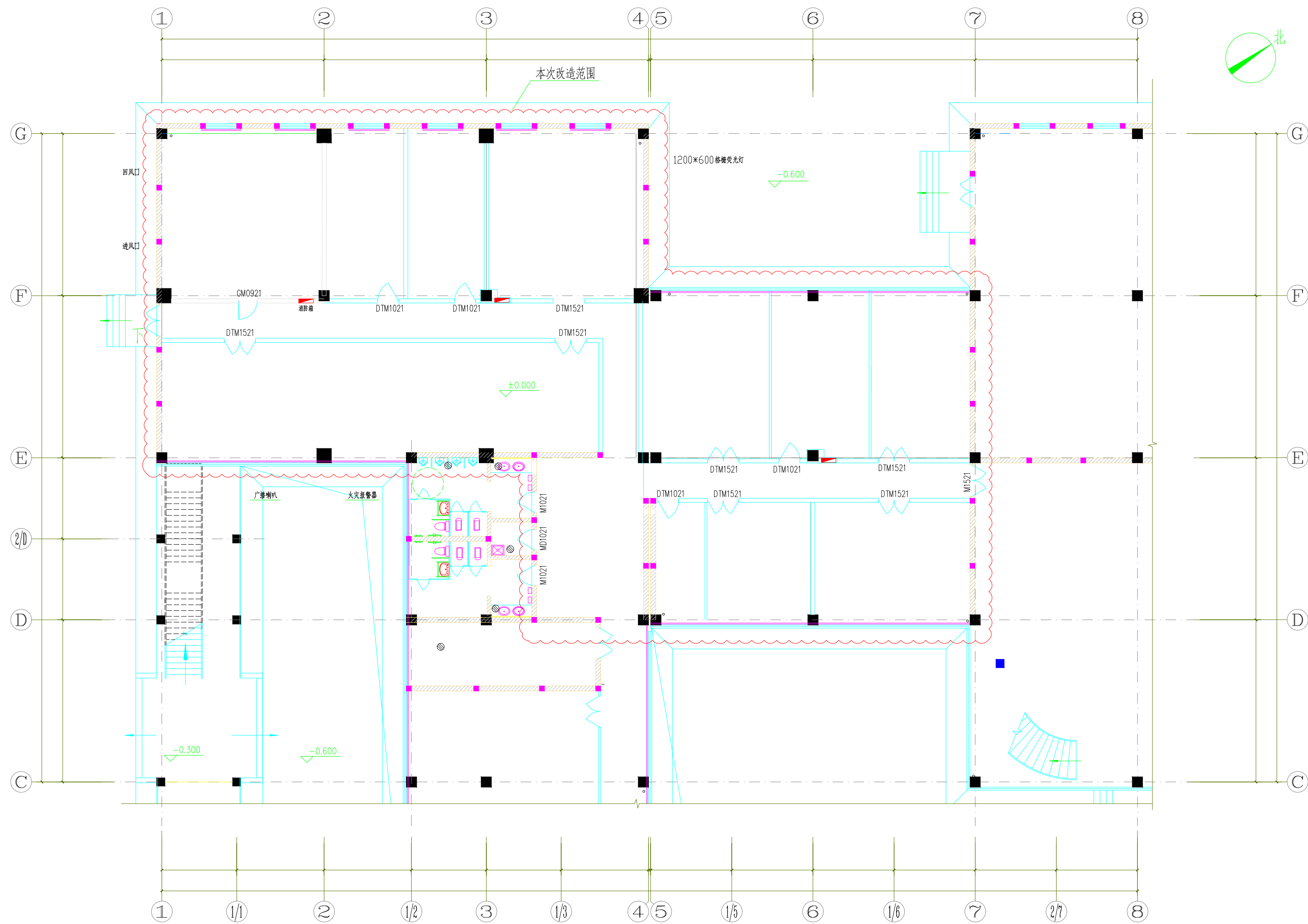
一层原始平面图
